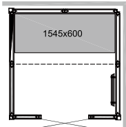
PANACEA 1717 1B Size: 1725×1725×2090mm 本体価格：4,345,000円
