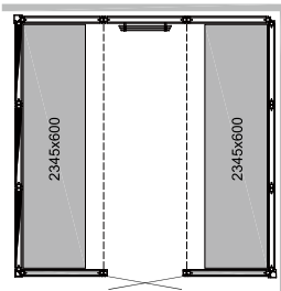
PANACEA 2525 2B Size: 2525×2525×2090mm 本体価格：7,810,000円
